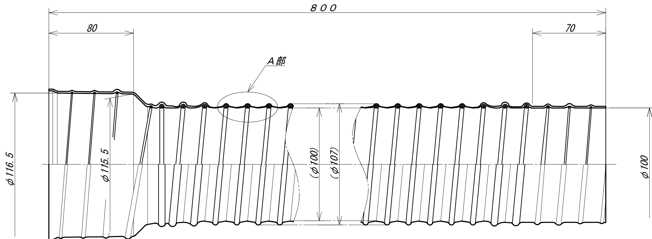
収縮時姿図 1 / 4
