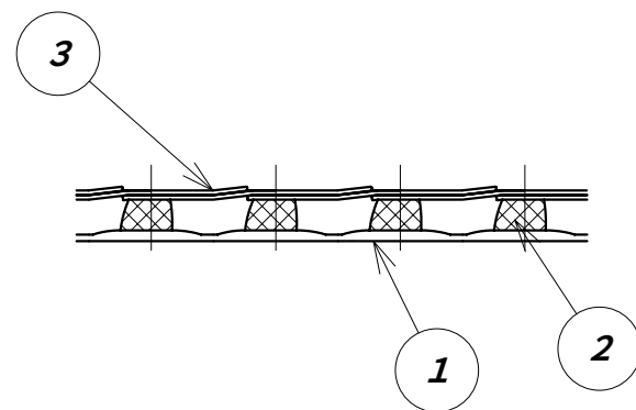
A部詳細 1/1
