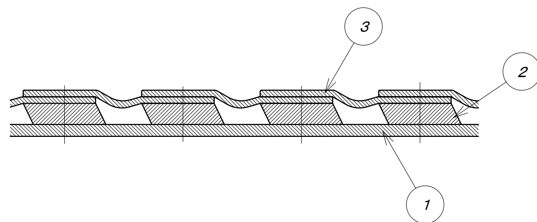
A部詳細
