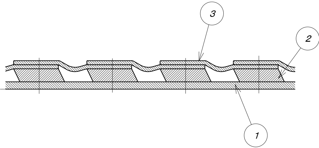
A部詳細
